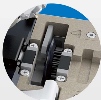
Auto-rotating blade
